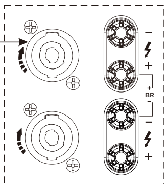
音箱螺旋插头 Speakon (NL4)
