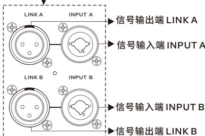
平衡XLR接线方式
