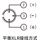
平衡XLR接线方式
